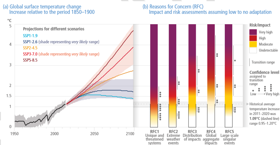
Figura 3-1. comparación entre Cambio de temperatura global media relativa a 1850-1900 y estimación de riesgo para distintos impactos bajo distintos escenarios futuros.
