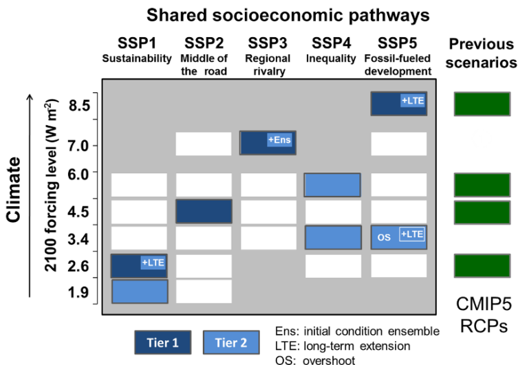
Figura 3-2. Interrelación entre trayectorias representativas de RCP y SSP en el marco del CMIP6
