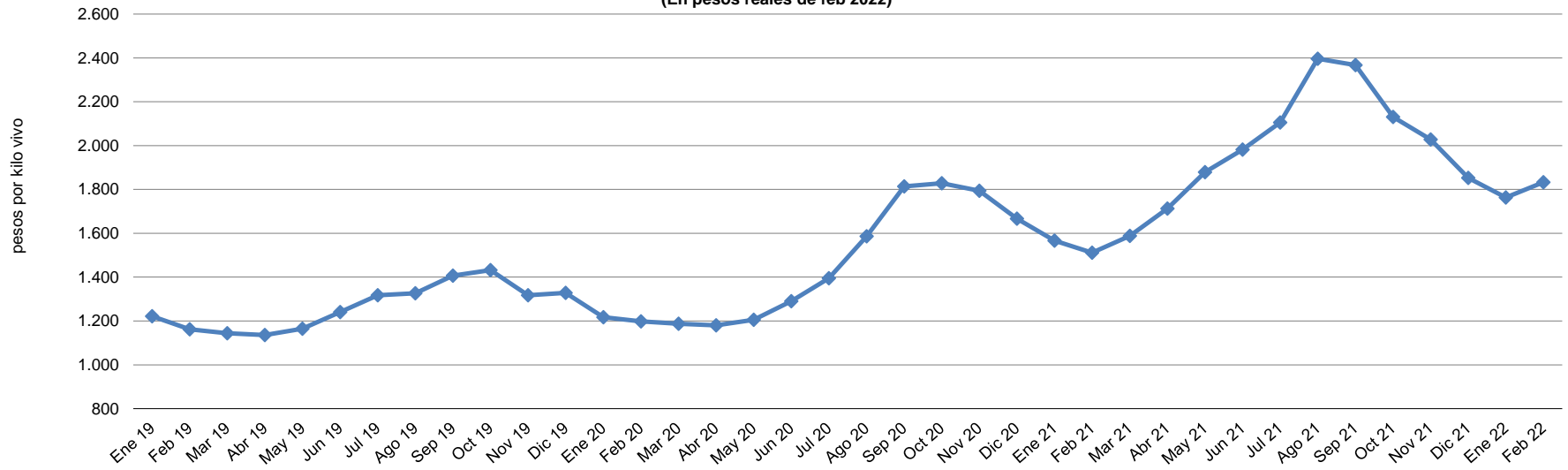
Gráfico 5 Precio promedio de novillo gordo a productor en la Región de Los Lagos Período ene 2019 - feb 2022 (En pesos reales de feb 2022)
