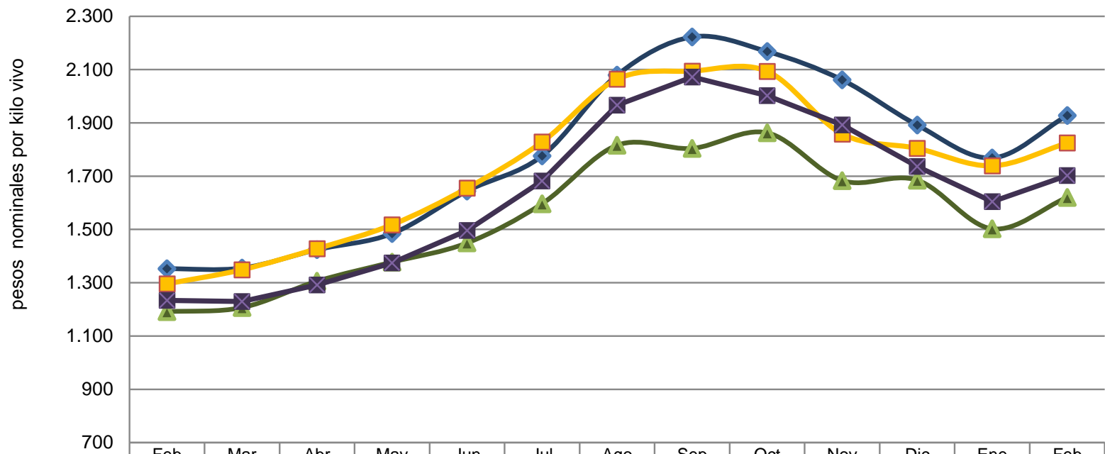
Gráfico 7 Precio nominal promedio nacional del ganado bovino para engorda y crianza Período feb 2021 - feb 2022 (Pesos de kilo vivo)
