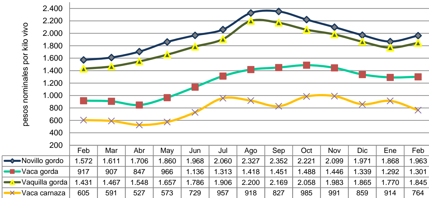
Gráfico 6 Precio nominal promedio nacional del ganado bovino para faena Período feb 2021 - feb 2022 (Pesos por kilo vivo)
