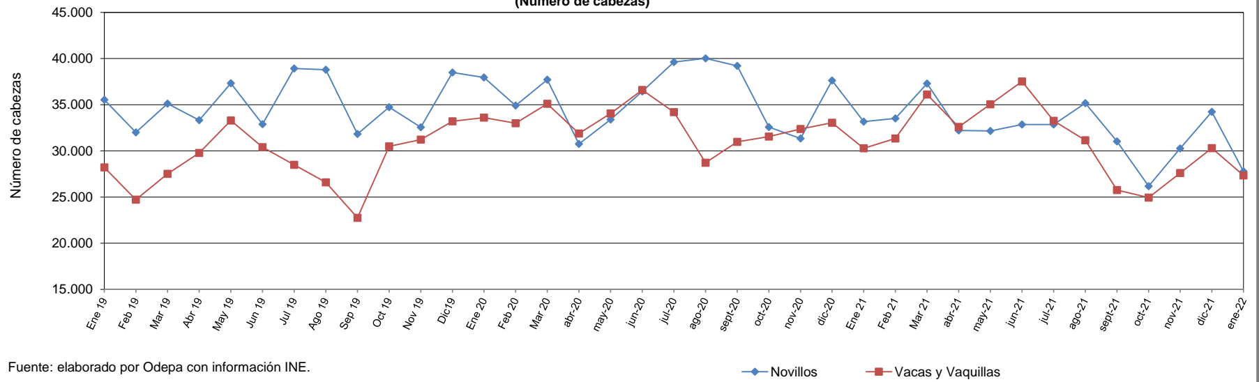
Gráfico 3 Beneficio de novillos y vacas y vaquillas Período Ene 2019- ene 2022 (Número de cabezas)
