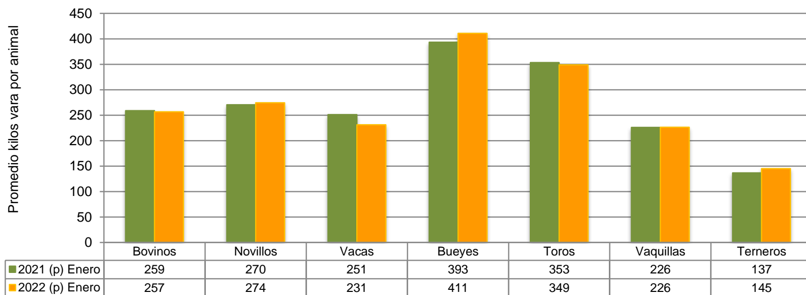
Gráfico 2 Peso promedio por categoría Periodo enero 2022 (Kilos en vara)
