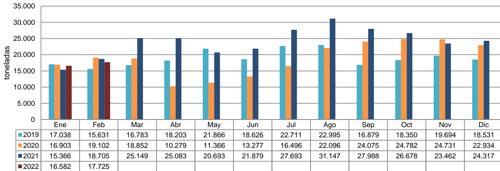
Gráfico 8 Importaciones mensuales de carne bovina Período ene 2019- feb 2022 (Toneladas)
