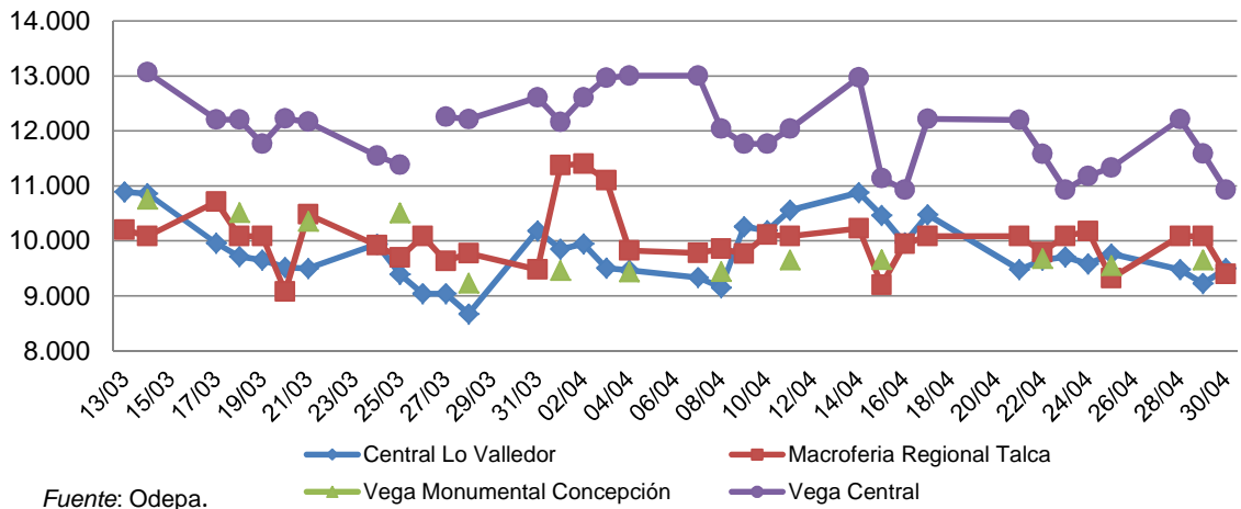
Gráfico 3 Precio diario de papa en los mercados mayoristas según mercado desde el 13 de marzo al 30 de abril de 2014 (en $/50 kilos sin IVA)
